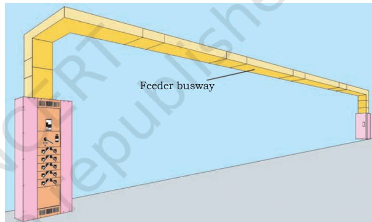
Fig. 2.9: Feeder busway
