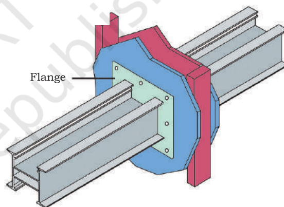
Fig. 2.31: Flange
